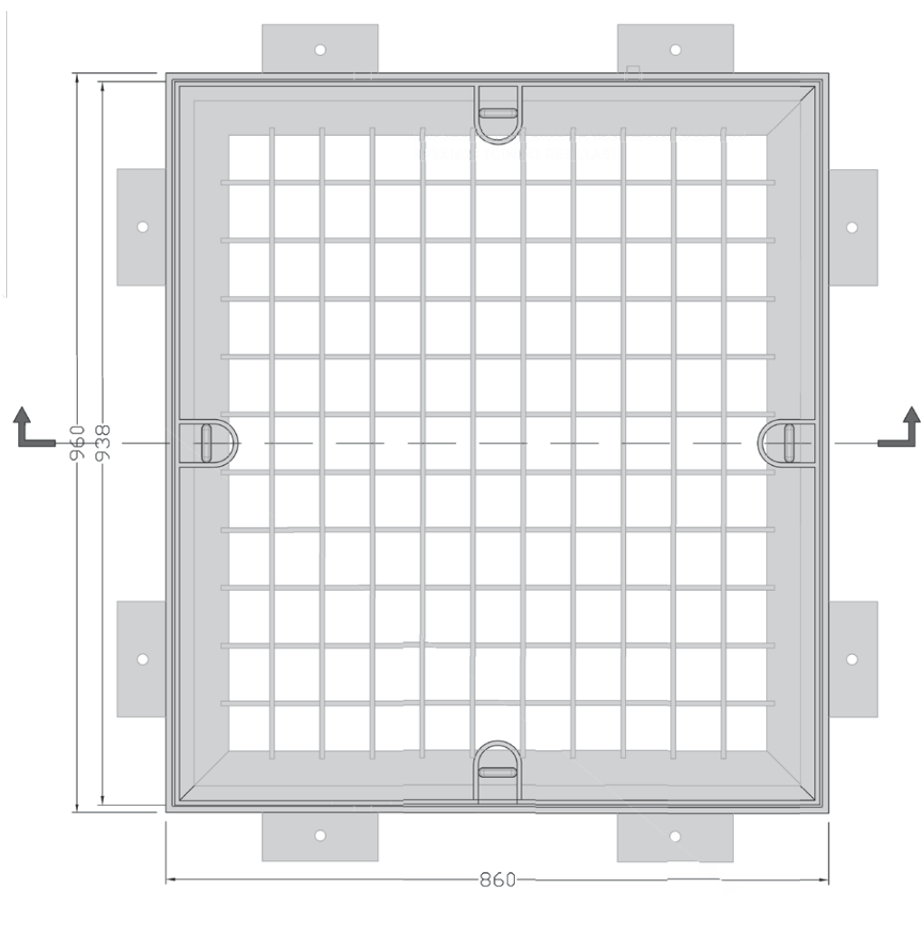
2210 - TAPA Y MARCO SIMPLE DM-2210 REV 7 VEREDA B125
